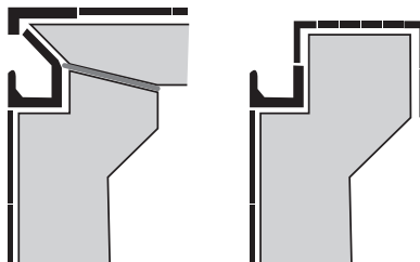
3.7. ábra: Vályúkialakítások. Balra sülyesztett vályú (balra) és nyitott vályú (jobbra) [3 p210]
