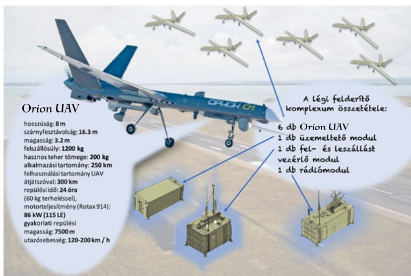
3. ábra: Az Orion UAV technikai paraméterei és a légi felderítő komplexum összetétele
