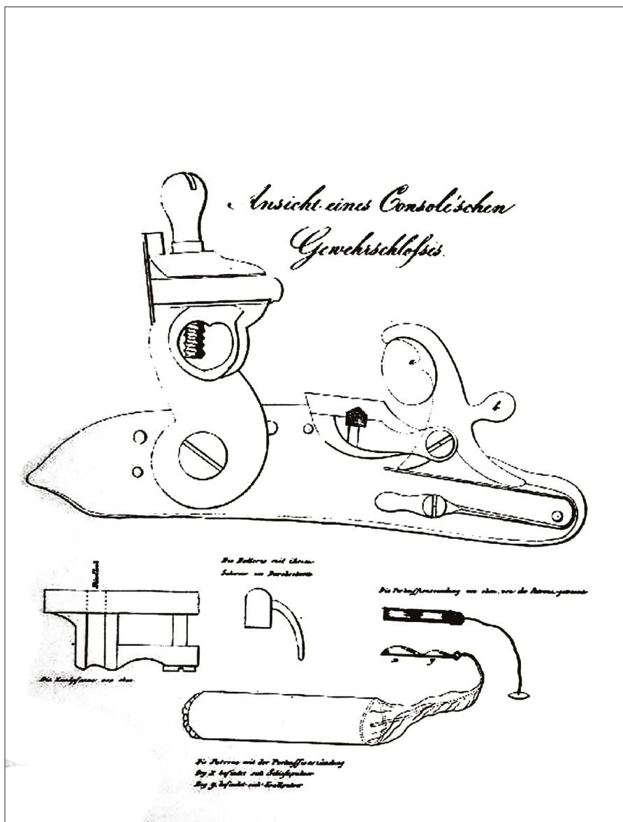
6. kép. Console-féle lakat és gyutaccsal ellátott töltény
