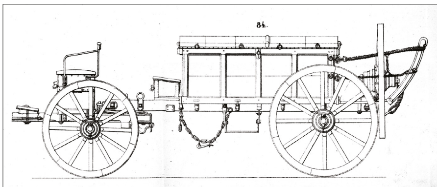
5. kép. A batfontos ütegben rendszeresített új típusú ütegcoksi
