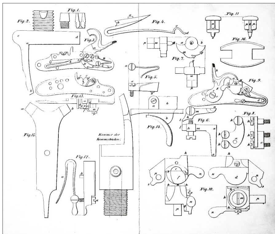
8. kép. Az Augustin-féle kis gépi gyutacsos lakat és a gyalogospuska alkatrészei Magyarázat: 1. mag; 2. csőfar; 3. a lakat belső oldala; 4. főrugó; 5. elsütő akasztó rugó; 6. elsütő akasztó; 7. dió; 8. bölcső; 9. a lakat külső oldala; 10. fedél; 11. fog; 12. fedélrugó; 13. lakatlemez serpenyővel; 14. ravasz; 15. csavarhúzó; 16. rugósatu)
